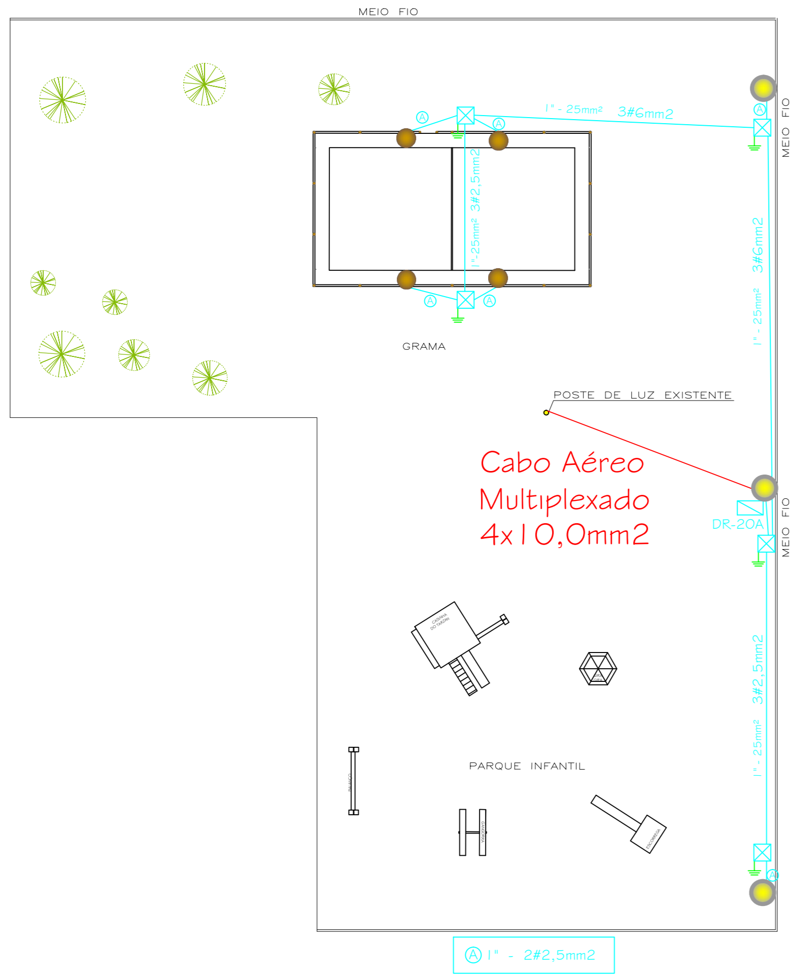
Planta Elétrica ESC.: 1/250
