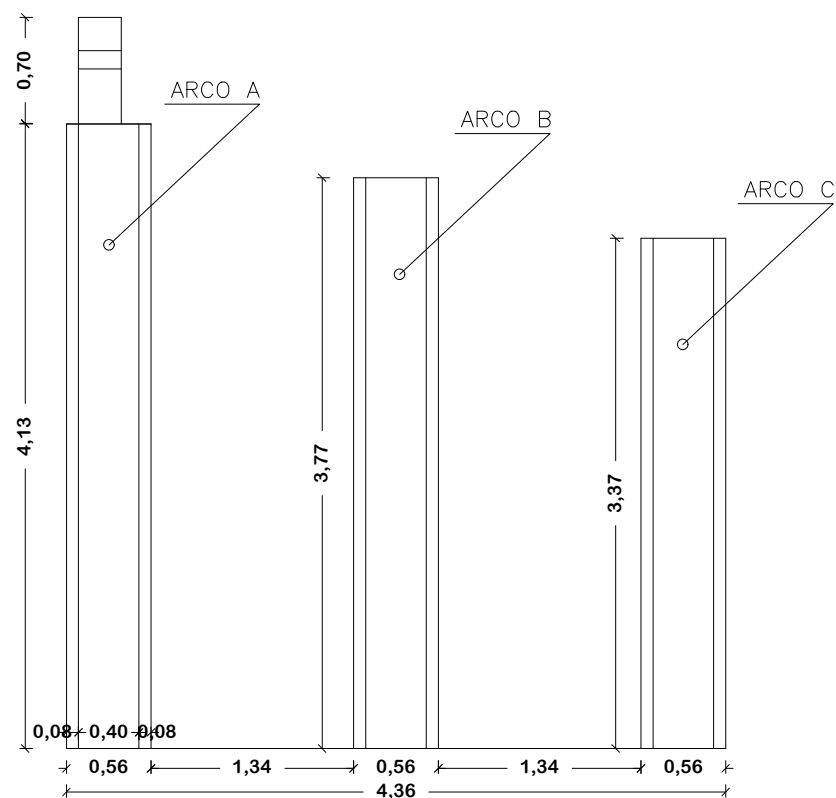
ESQUEMA LATERAL – ARCOS ESC. 1/50
