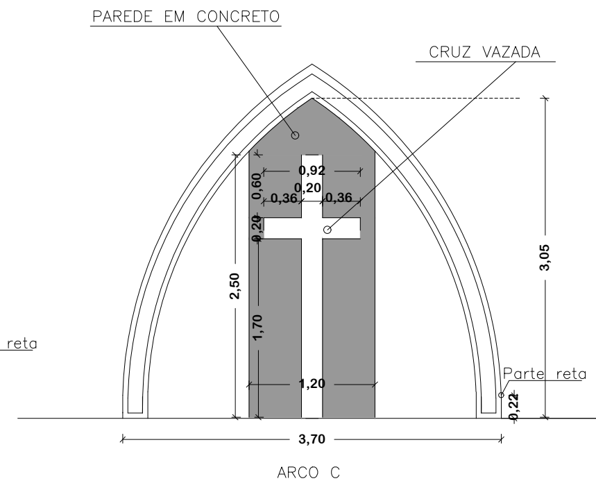
ESQUEMA FRONTAL – ARCOS ESC. 1/50
