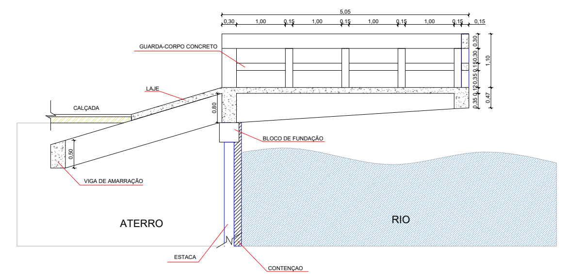
CORTE PLATAFORMA ESCALA: 1/75
